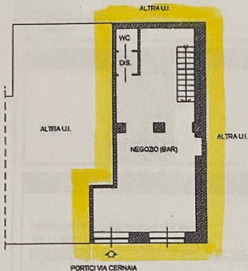
PIANTA PIANO TERRENO 1° f.t. - H=4.40 mt
