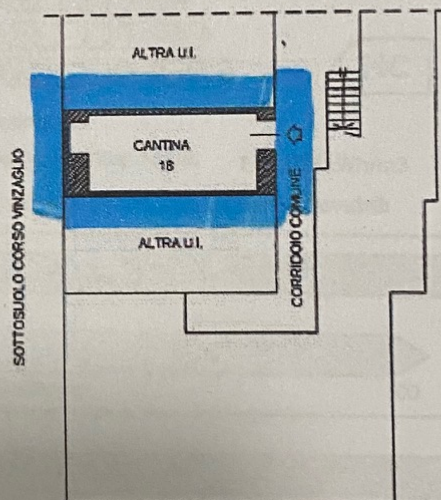
PIANTA PIANO INVERNOTTI - Hm=2.45 mt
