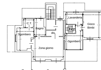
PIANTA PIANO PRIMO (2 f.t.) Stato di Fatto H = 2,40 mt
