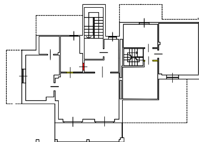
PIANTA PIANO PRIMO (2 f.t.) Sovrapposizioni H = 2,40 mt
